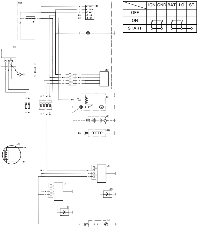
Tipo con bobina de carga de 2,7 A y con caja de control
