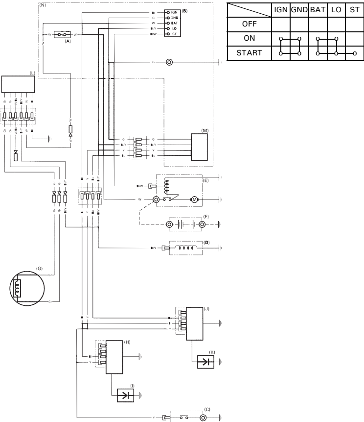
Tipo con caja de control y bobina de carga de 17A
