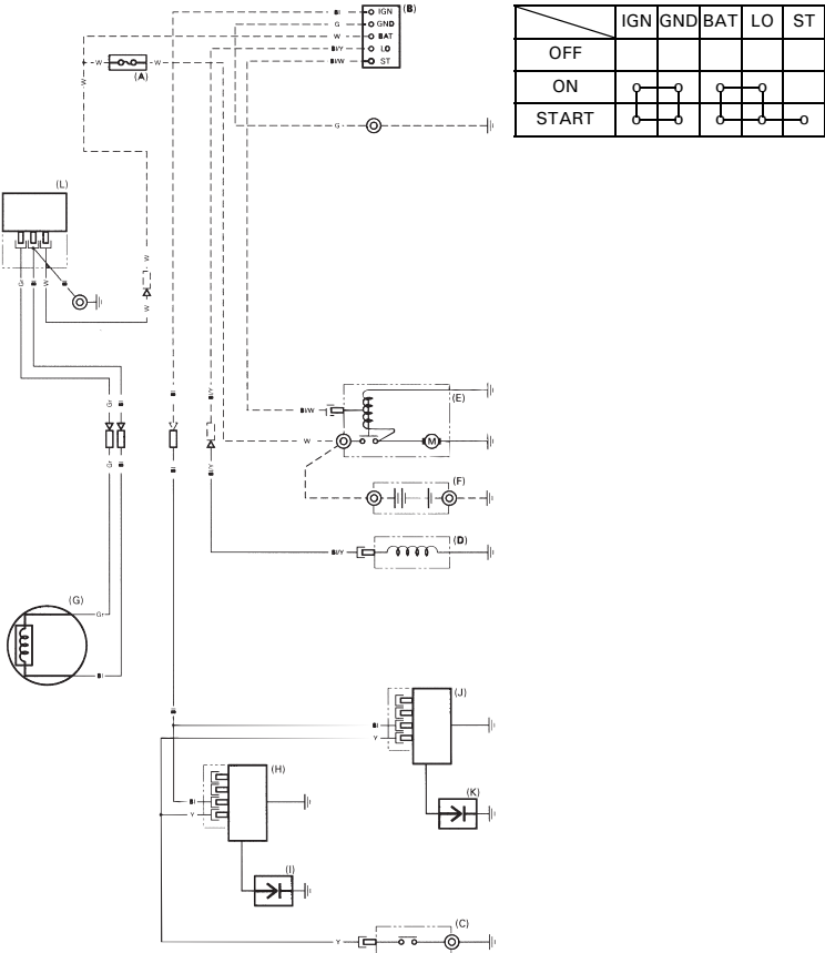
Tipo con bobina de carga de 2,7 A y sin caja de control
