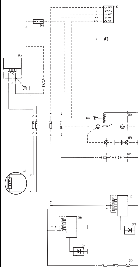
Type bobine de charge 2,7 A et sans boîtier de commande
