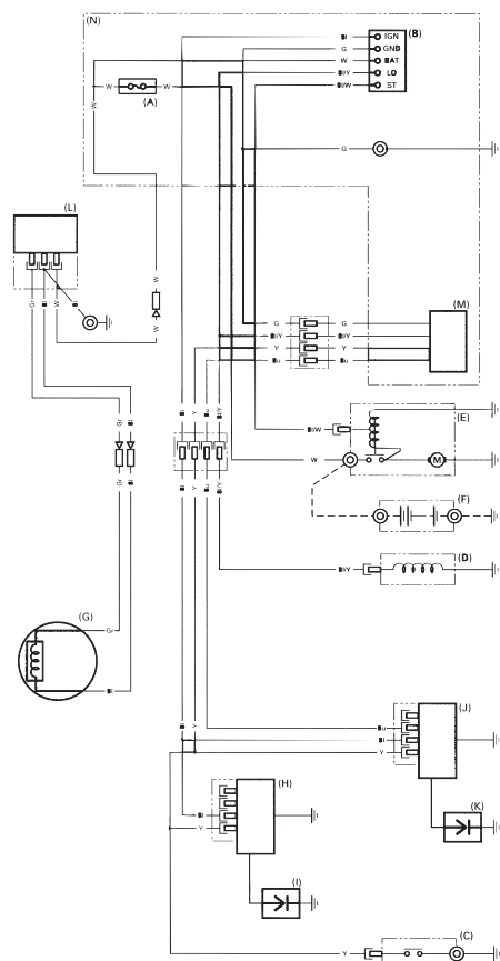
Type bobine de charge 2,7 A et avec boîtier de commande
