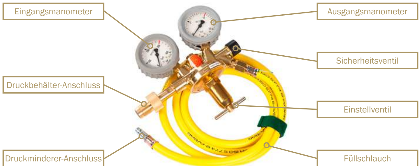
Abbildung 7.2: Druckminderer
