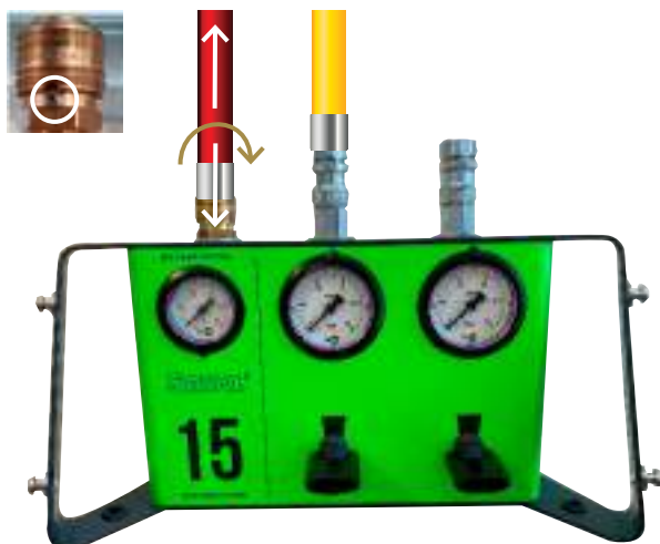
Abbildung 7.14: Den Füllschlauch vom Steuerorgan abtrennen
