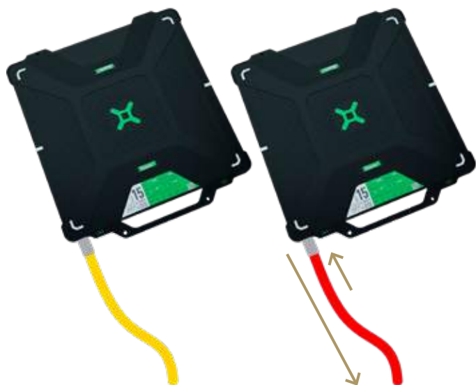
Abbildung 7.16: Die Verbindungsschläuche vom Hebekissen abtrennen
