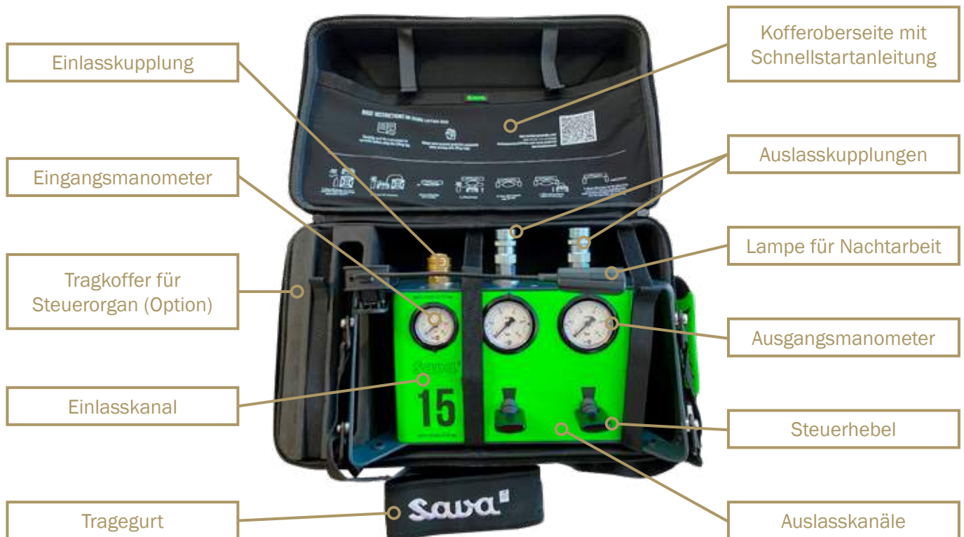
Abbildung 7.5: EXP-Steuerorgan
